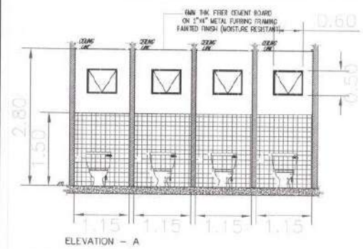
ELEVATION - A
