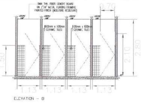
ELEVATION - B
