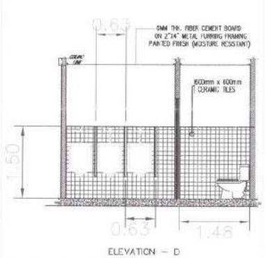
ELEVATION - D
