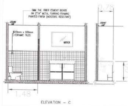
ELEVATION - C
